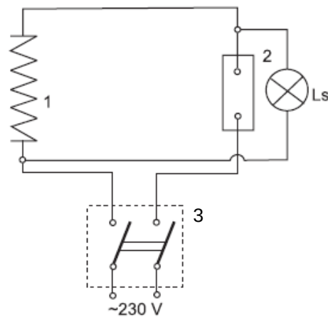
Rys.3 Schemat elektryczny ogrzewacza
