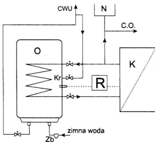
Rys.4 Schematy przyłączeniowe ogrzewaczy do instalacji C.O.
