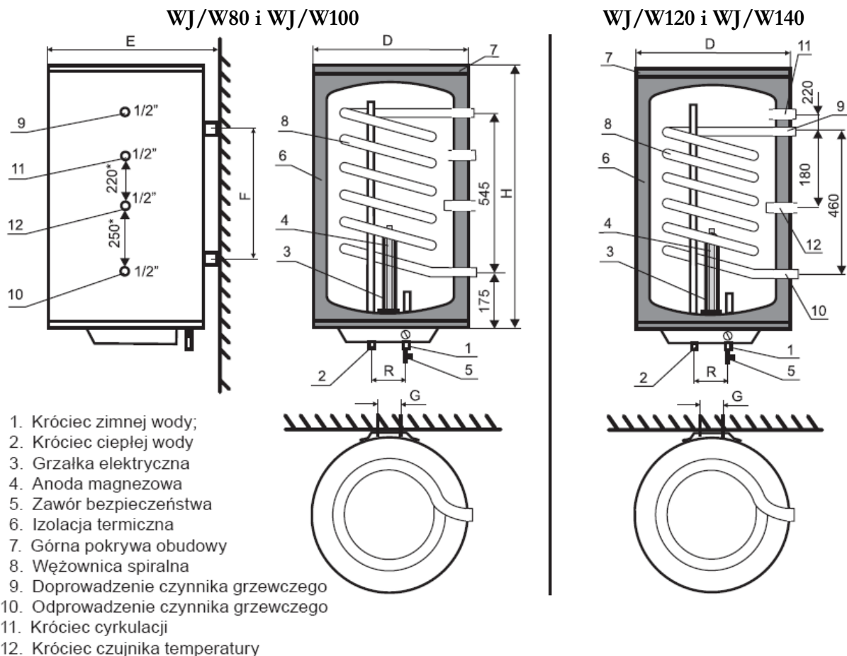
Rys.1 Budowa i wymiary gabarytowe ogrzewaczy WJ/W DELFIN-plus
