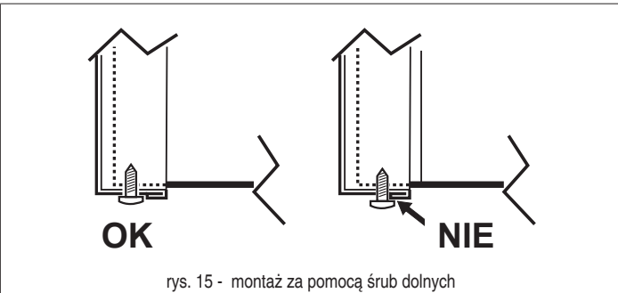
rys. 15 - montaż za pomocą śrub dolnych
