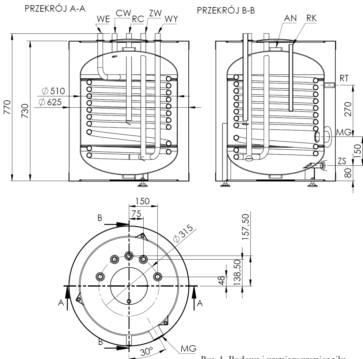
Rys. 1 Budowa i wymiary wymiennika KELLER 100/MG
